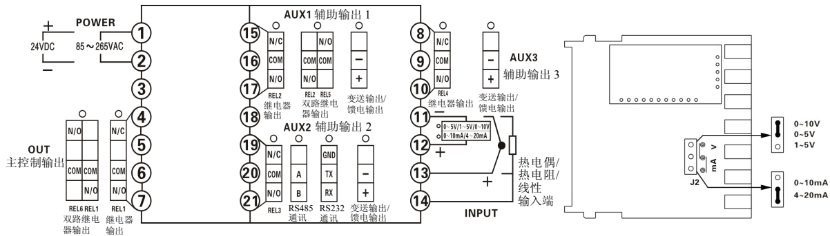
F 型接线图
