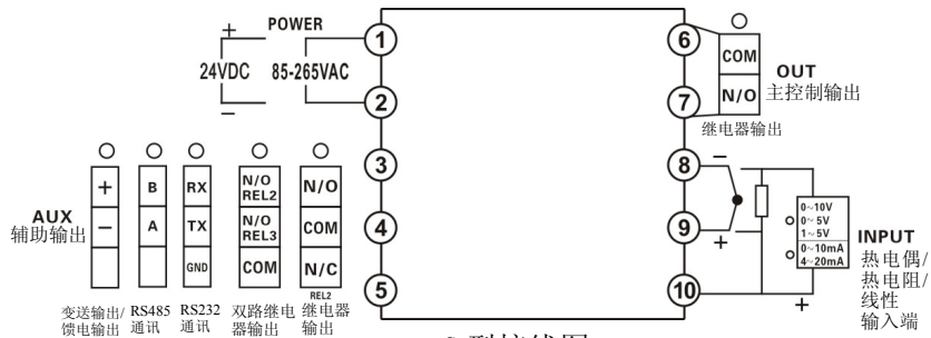
G 型接线图
